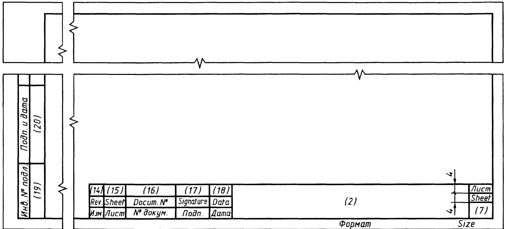
Форма 3 — Основная надпись для текстовых конструкторских документов (последующие листы)
