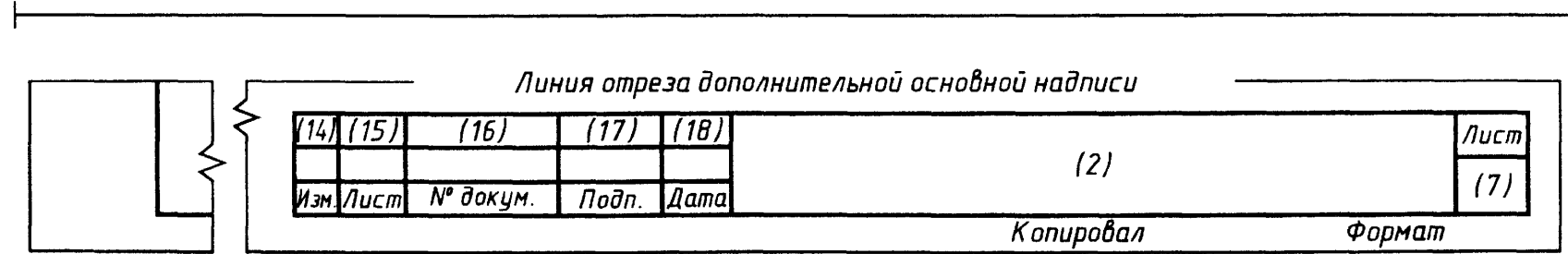
Форма 4 — Основная надпись на чертежи
